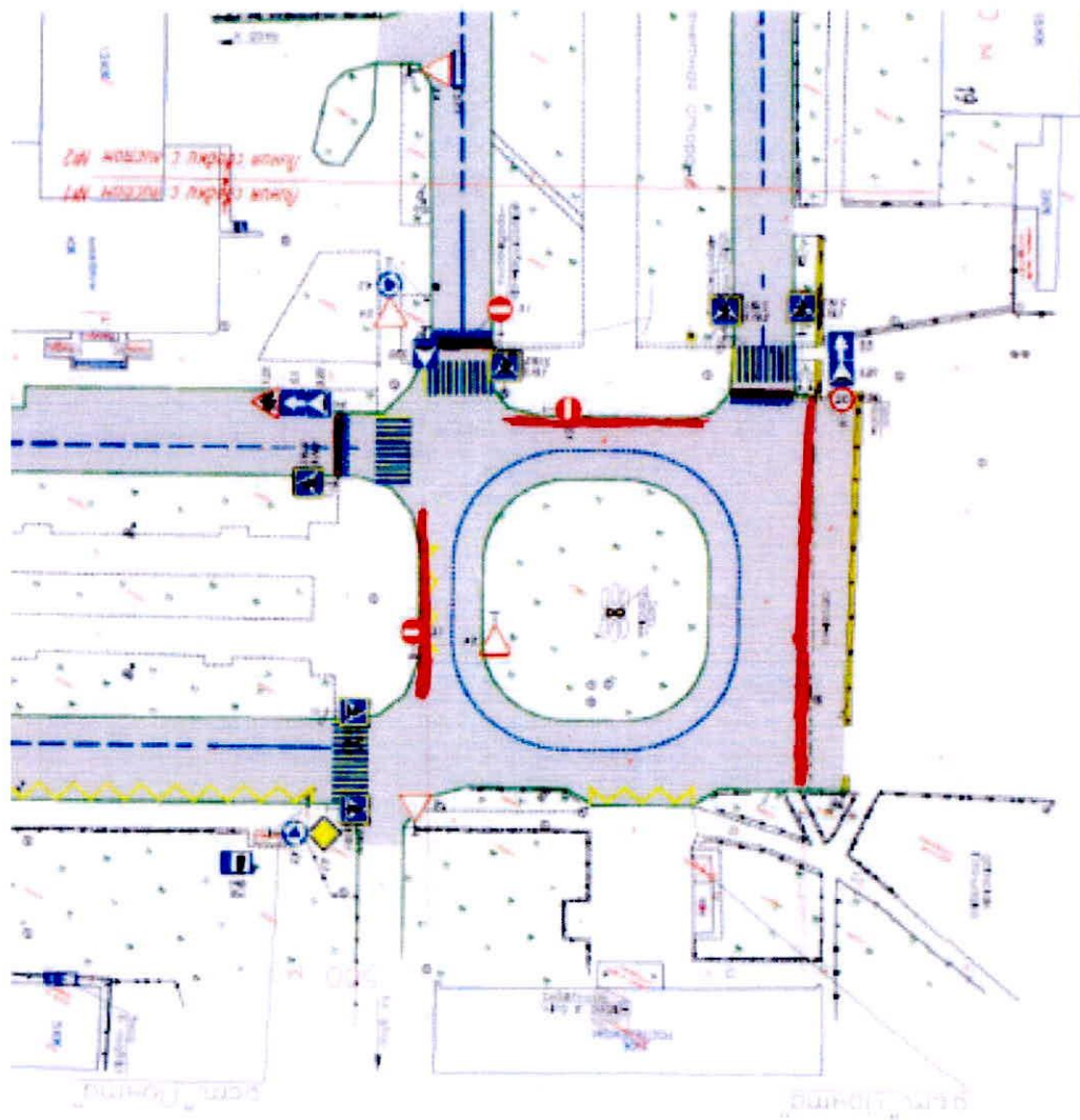
15. Схема участков для установки дорожных знаков 3.27 «Стоянка запрещена» с дополнительными знаками 8.24 «Работает эвакуатор», ограничивающих стоянку и парковку автомобилей на пересечении бульваров №1 и №2 в 1 микрорайоне, поселение Московский.
