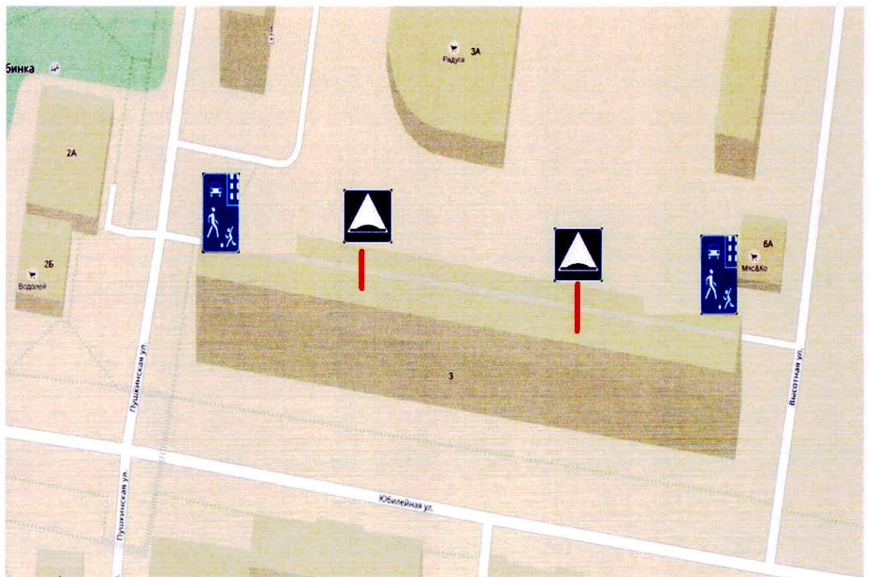
38. Схема установки ИН и дорожных знаков 5.21 «Жилая зона» по адресу: ул. Юбилейная д. 3, городской округ Щербинка.
