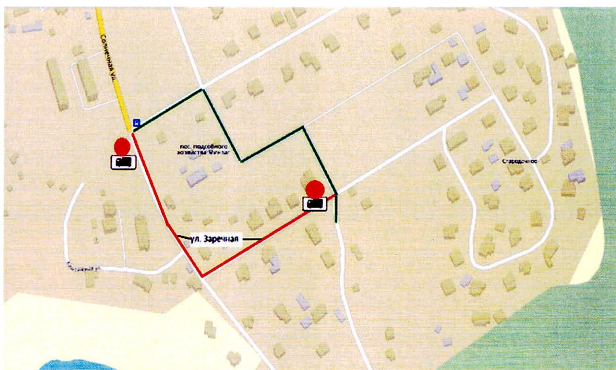
11. Схема установки дорожного знака 3.4 «Движение грузовых автомобилей запрещено» по ул. Заречной в пос. Минзаг, поселение Краснопахорское.
