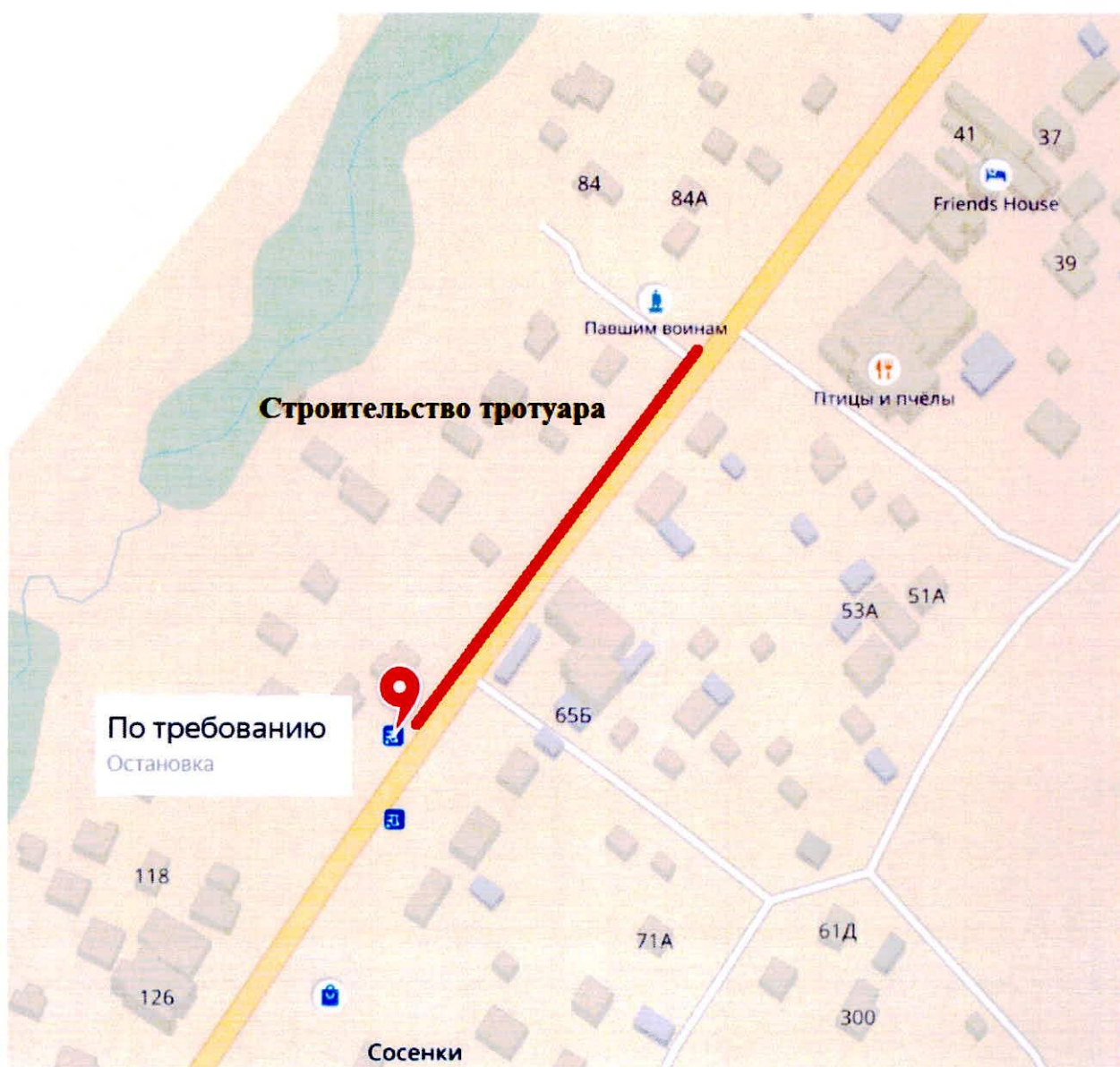
24. Схема обустройства тротуаров и подходов к пешеходному переходу в д. Сосенки, вблизи остановки «По требованию», поселение Сосенское.
