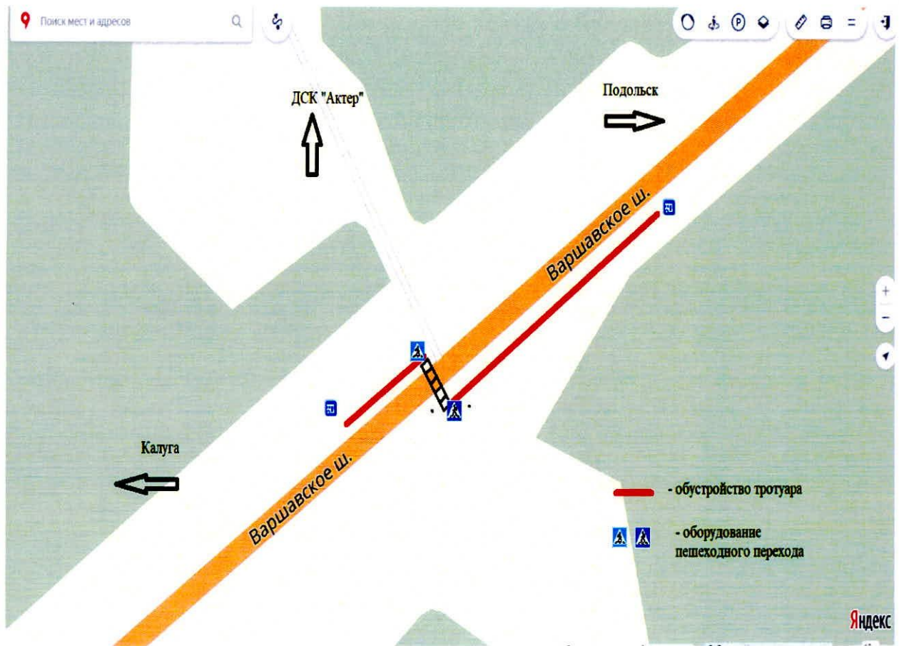
5. Схема организации пешеходного перехода на Варшавском шоссе, между остановочными площадками «Баранково», поселение Вороновское.
