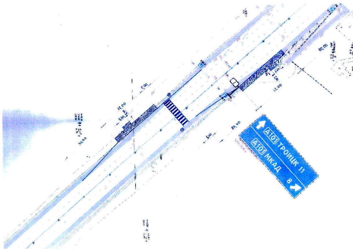
Схема организации остановок общественного транспорта с регулируемым пешеходным переходом вблизи ЖК «Фестиваль», пос. Сосенское.
