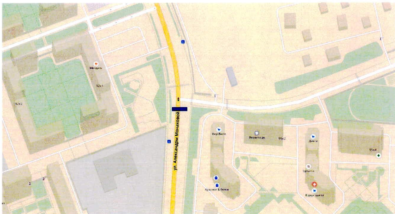
Схема организации пешеходного перехода на ул. Александры Монаховой у д. 95 к.1, пос. Сосенское.
